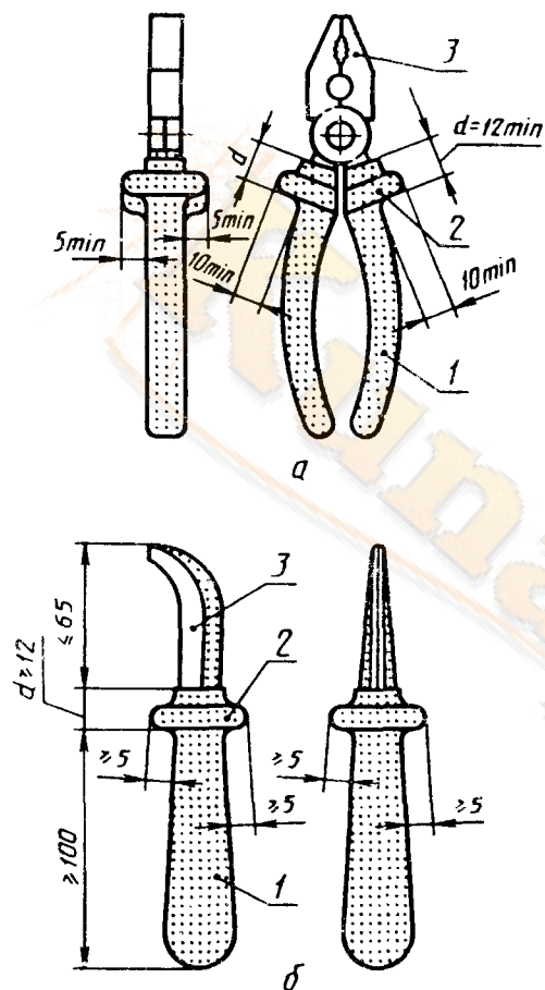
Рисунок 2 — Типы изоляции пассатижей (а) и ножей (б)
