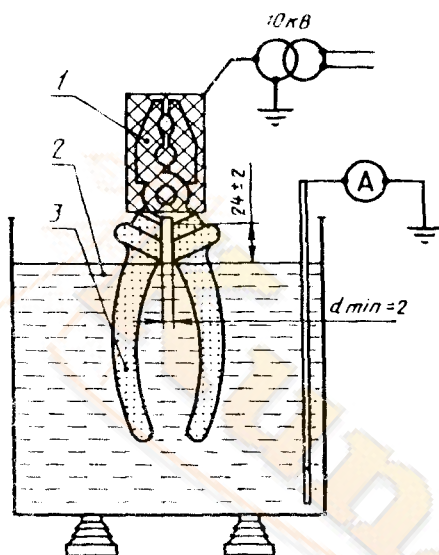
Рисунок 5 — Оборудование для электрического испытания и изолированных инструментов
