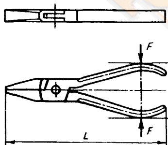
Рисунок 12 — Изолирующие плоскогубцы. Испытание рукояток на изгиб
